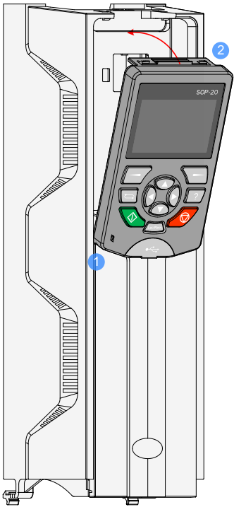
Рисунок 3-1 Установка панели SOP-20-880 на переднюю крышку блока HCU
