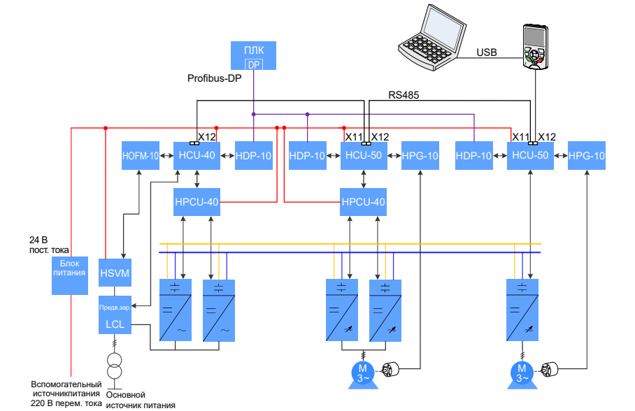
Рисунок 3-6 Пример организации сети для панели SOP-20-880
