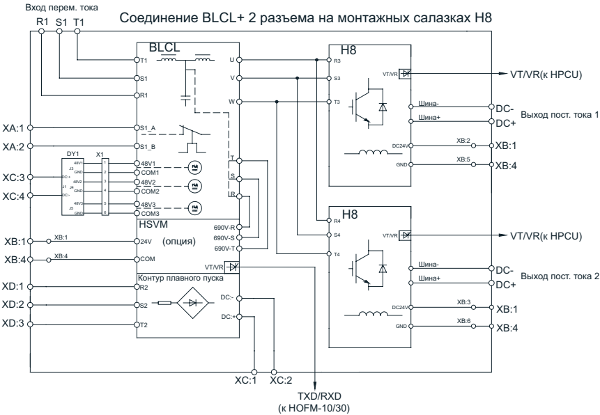
Рис. 3-15 Разъемы на монтажных салазках BLCL+2H8
