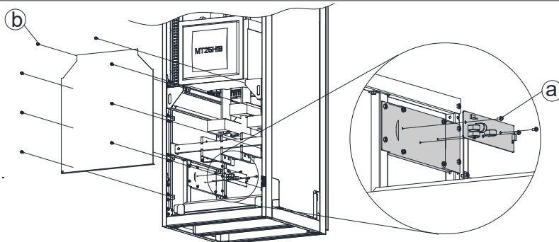
Рис. 5-7 Замена платы молниезащиты
