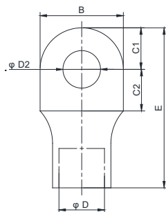
Рис. 3-17 Внешний вид наконечника
