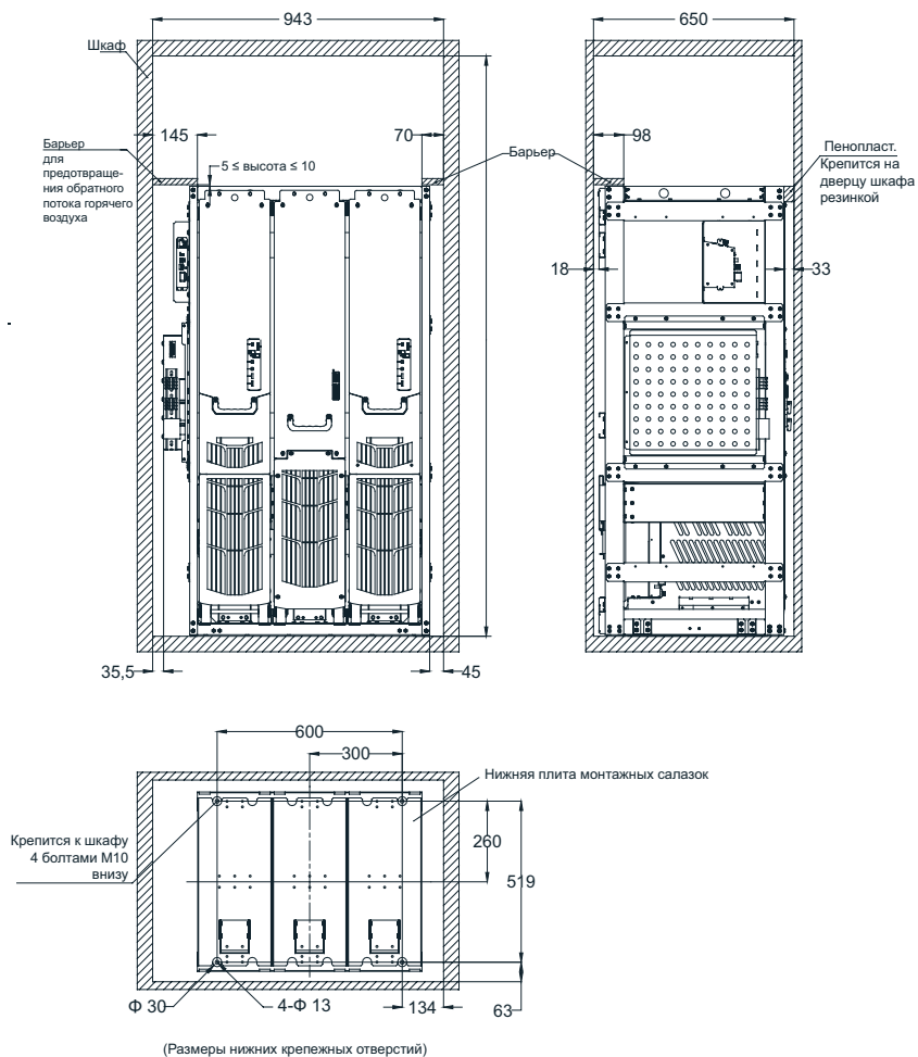
Рис. 2-13 Минимальные требования к размерам шкафа (мм)
