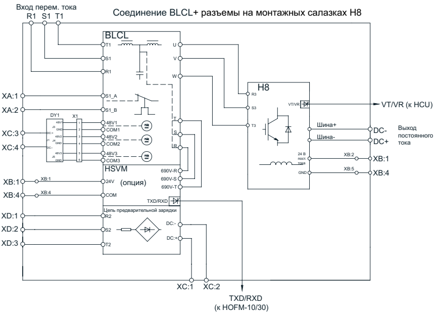
Рис. 3-13 Разъемы на монтажных салазках BLCL+H8
