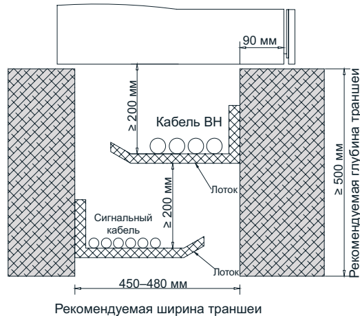
Рис. 2-24 Компоновка основания
