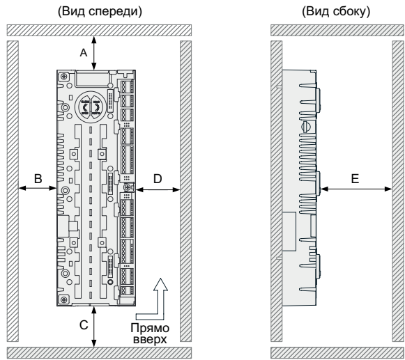
Рис. 4-4 Пространство для монтажа (в мм)
