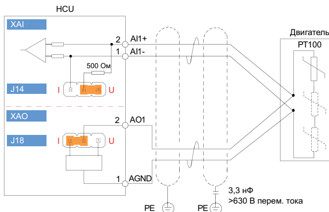
Рис. 4-11 Измерение температуры с использованием AI и АО
