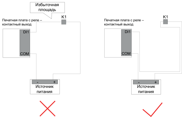
Рис. 3-6 Прокладка кабелей без большой площади петли
