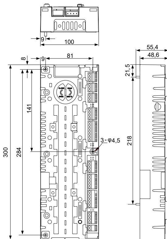
Рис. 4-3 Размеры HCU (в мм)
