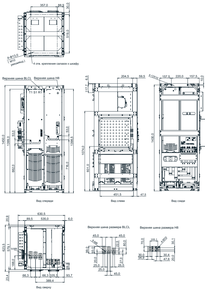
Рис. 1-11 Размеры монтажных салазок активного выпрямителя BLCL+H8 (мм)
