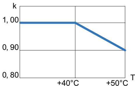
Рис. 1-19 Температура окружающей среды
