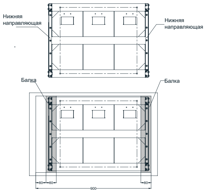
Рис. 2-14 Размеры нижних балок (мм)
