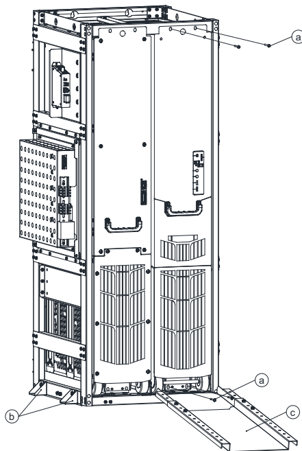
Рис. 2-9 Извлечь модуль Н8 из монтажных салазок.
