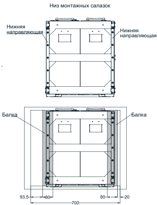
Рис. 2-8 Размеры балки (мм)
