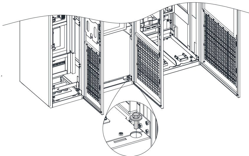
Рис. 2-28 Крепление шкафа
