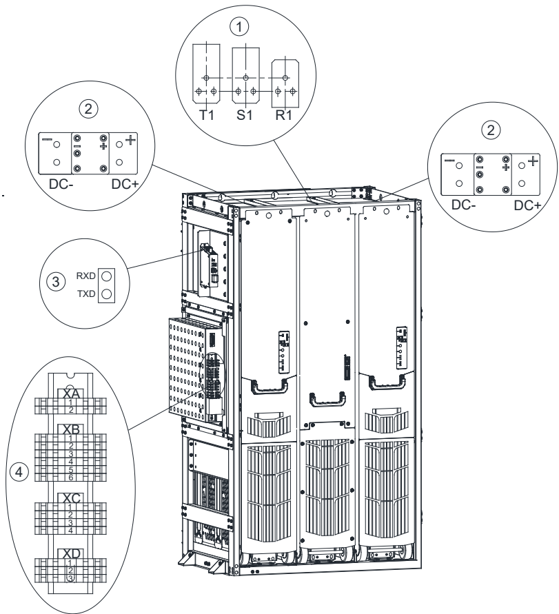
Рис. 3-14 Разъемы на монтажных салазках BLCL+2H8
