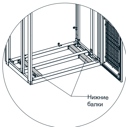
Рис. 2-7 Нижние балки
