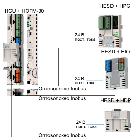
Рис. 4-10 Пример подключения HESD
