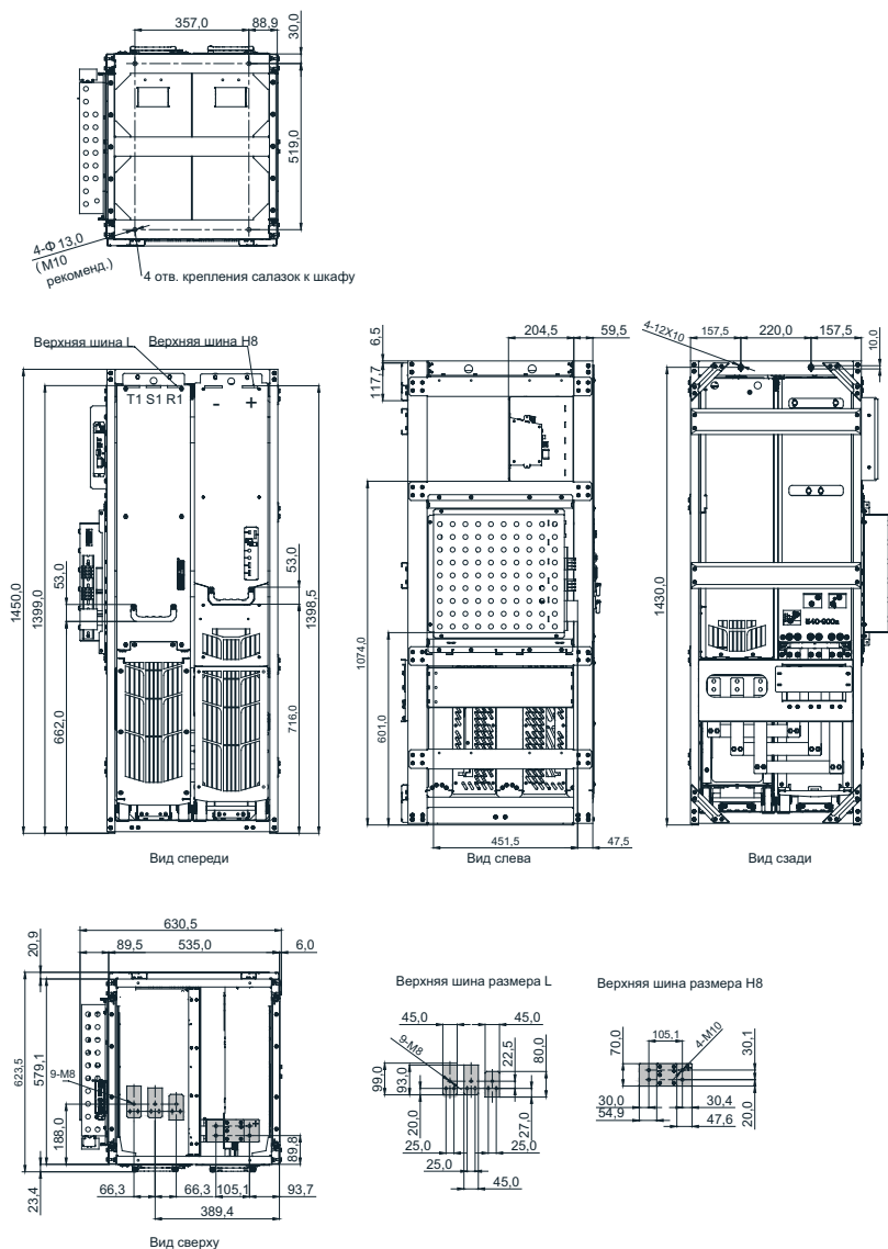
Рис. 1-11 Размеры монтажных салазок рекуперативного выпрямителя L+H8 (мм)
