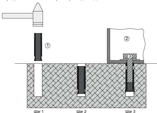
Рис. 2-14 Монтаж анкеров
