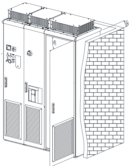
Рис. 2-12 Пространство, предусмотренное для открытия/закрытия дверцы (в мм)
