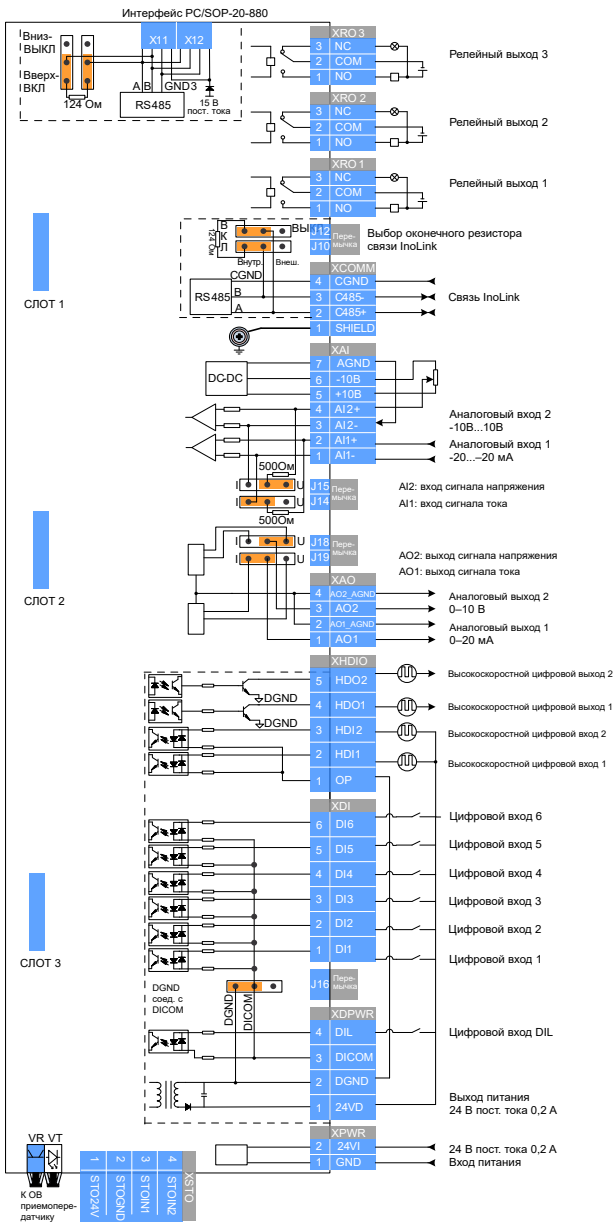
Рис. 4-6 Клеммы модуля управления НСУ
