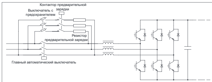
Рис. 3-18 Предварительная зарядка конденсатора шины постоянного тока
