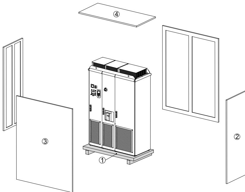
Рис. 2-16 Распаковка изделия
