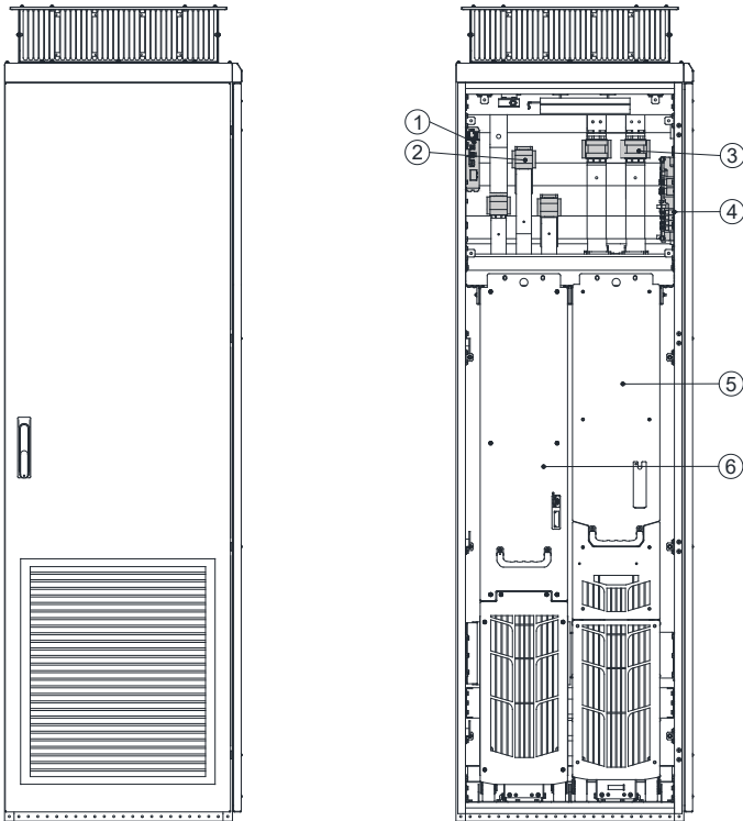
Рис. 1-17 Компоновка шкафа рекуперативного выпрямителя (L+H8)
