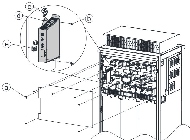
Рис. 5-6 Замена HSVM-10
