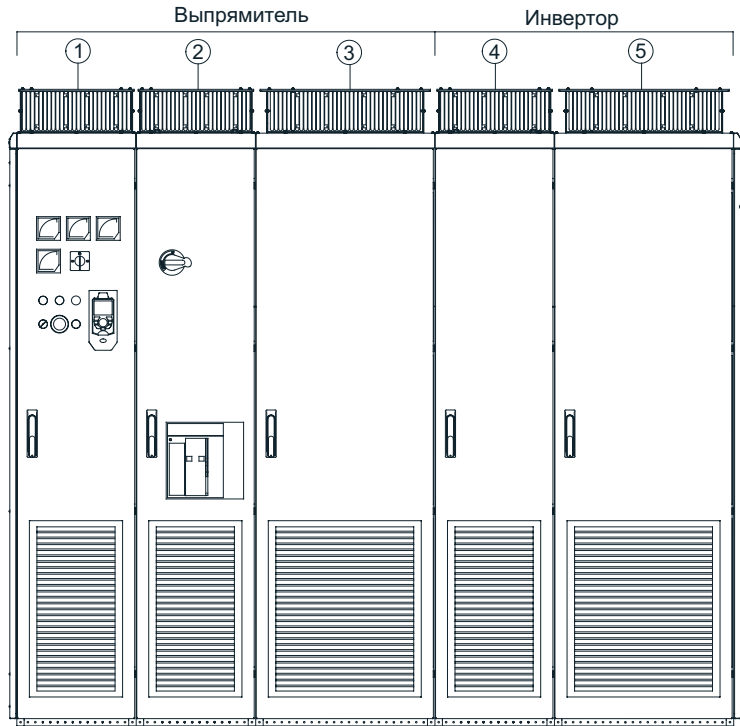
Рис. 1-14 Компоновка рекуперативного выпрямителя и системы привода
