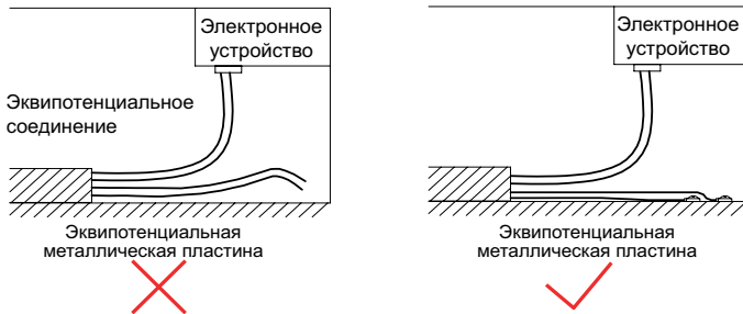
Рис. 3-5 Обращение с неиспользуемыми жилами в многожильных кабелях
