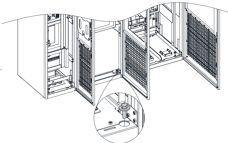
Рис. 2-19 Крепление шкафа
