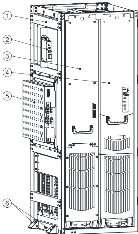
Рис. 1-10 Монтажные салазки рекуперативного выпрямителя L+H8
