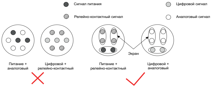
Рис. 3-4 Прокладка многожильных кабелей
