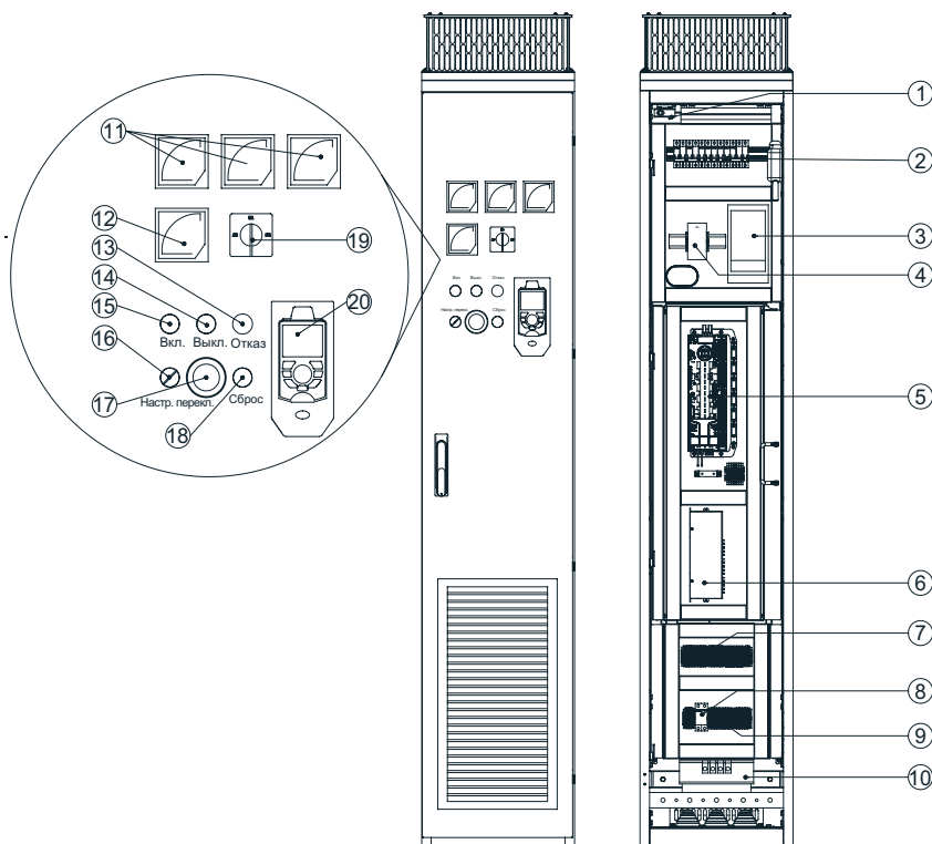
Рис. 1-15 Компоновка шкафа вспомогательного оборудования
