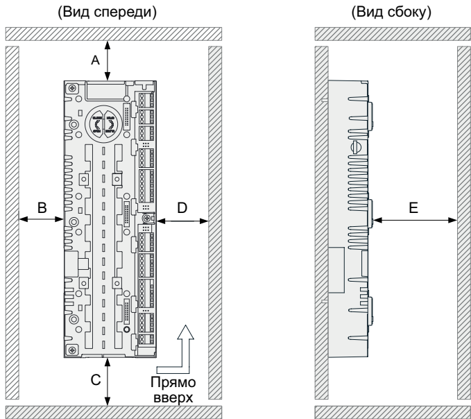
Рис. 4-4 Пространство для монтажа
