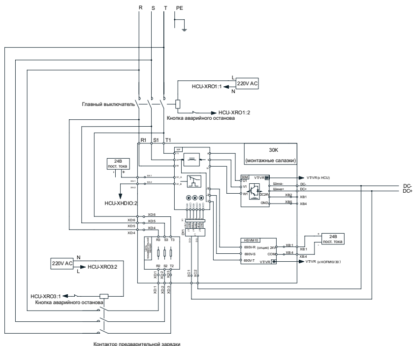
Рис. 3-19 Типовой электромонтаж шкафа
