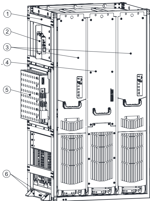
Рис. 1-12 Монтажные салазки рекуперативного выпрямителя L+2H8
