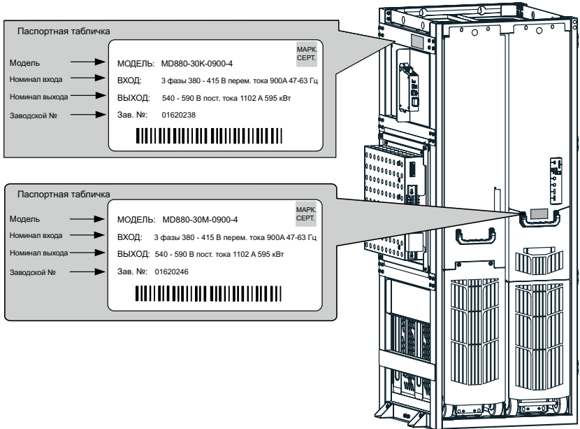
Рис. 1-1 Паспортная табличка
