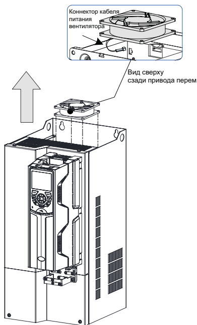
Рис. 5-17 Отсоединение кабеля питания
