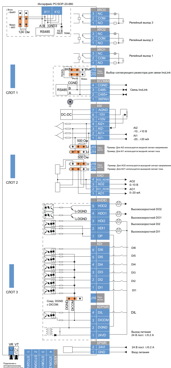
Рис. 4-6 Клеммы модуля управления HCU
