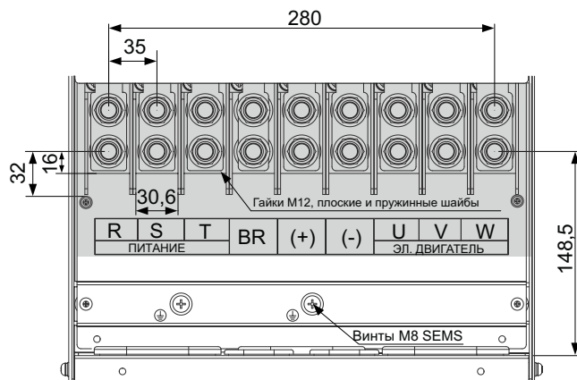
Рис. 3-30 MD880-01S-0183-4-B/MD880-01S-0217-4/MD880-01S-0262-4
