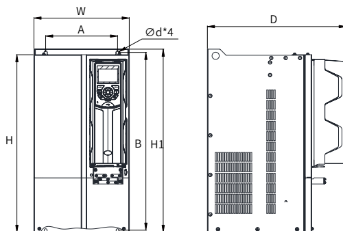
Рис. 1-7 Габаритные и монтажные размеры конструкций T2 - T9
