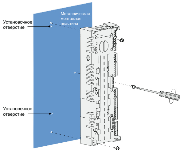
Рис. 4-4 Монтаж HCU
