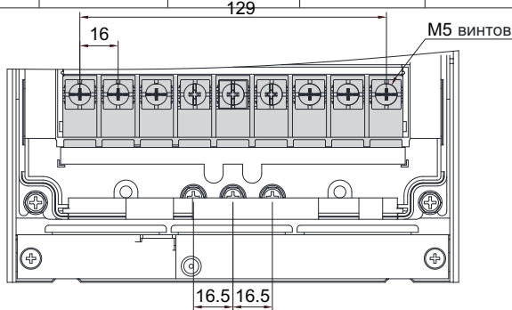
Рис. 3-26 MD880-01S-0038-4-B
