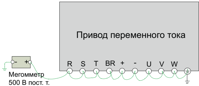
Рис. 5-14 Проверка изоляции на главной цепи
