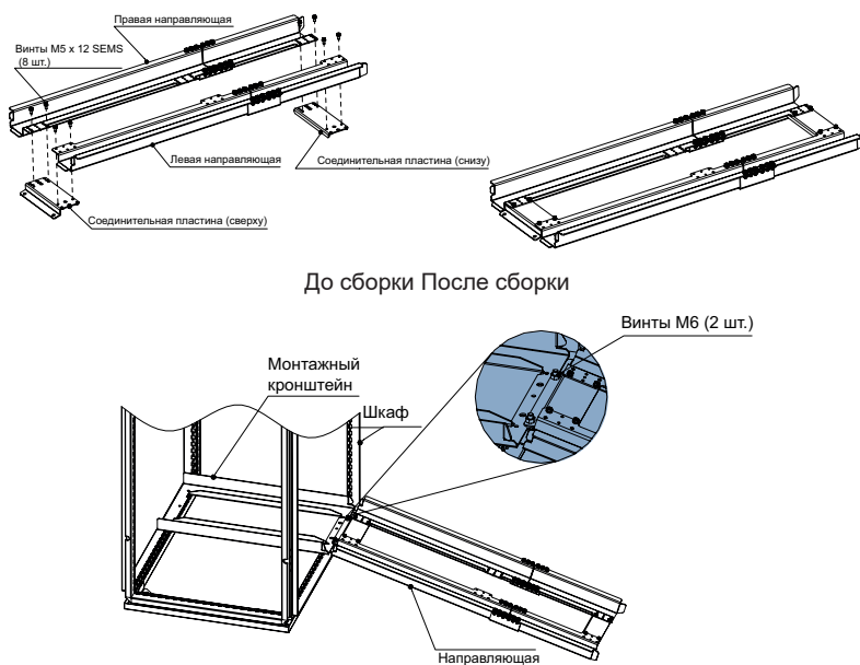
Рис. 2-16 Сборка направляющей в шкафу
