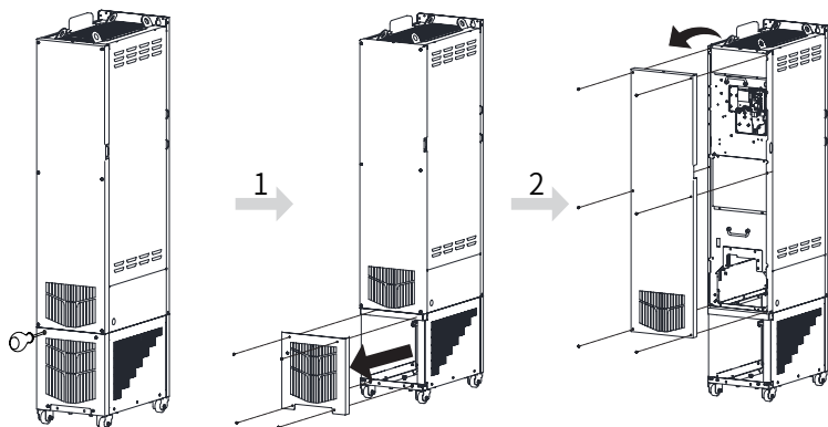
Рис. 2-25 Снятие крышек конструкций T10 - T12
