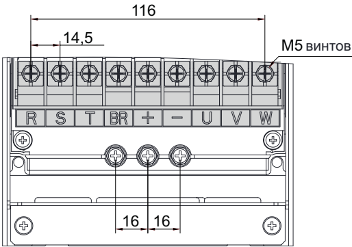
Рис. 3-25 MD880-01S-0024-4-B/MD880-01S-0033-4-B
