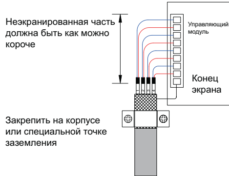
Рис. 3-9 Требования к экранированным кабелям питания
