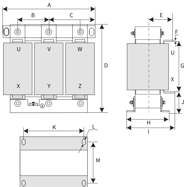
Рис. 6-29 Размеры выходного реактора переменного тока 150 - 250 A
