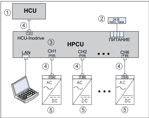
Рис. 4-8 Электрические соединения
