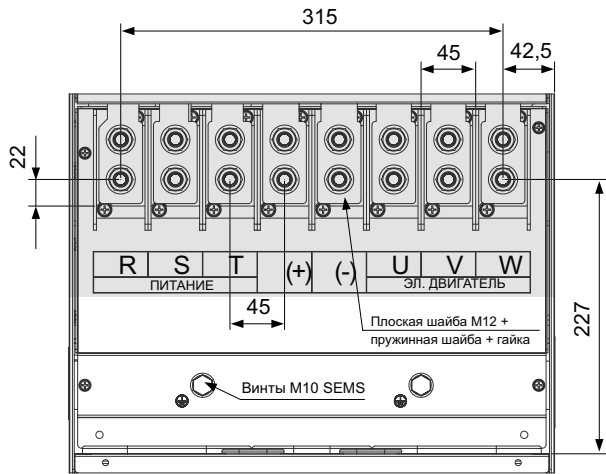
Рис. 3-31 MD880-01S-0314-4/MD880-01S-0383-4
