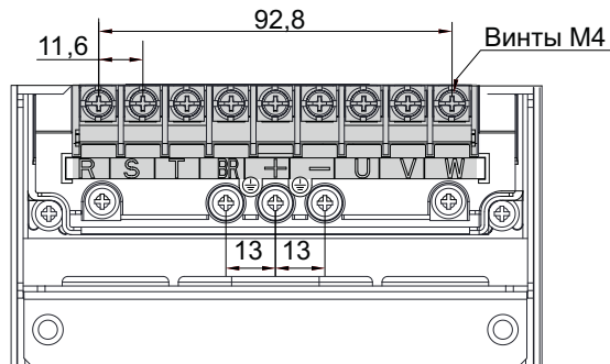
Рис. 3-24 MD880-01S-0012-4-B/MD880-01S-0017-4-B
