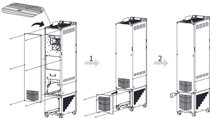
Рис. 2-26 Установка крышек конструкций T10 - T12
