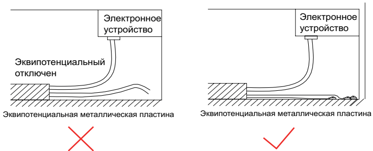
Рис. 3-6 Действия с оставшимися жилами в многожильных кабелях
