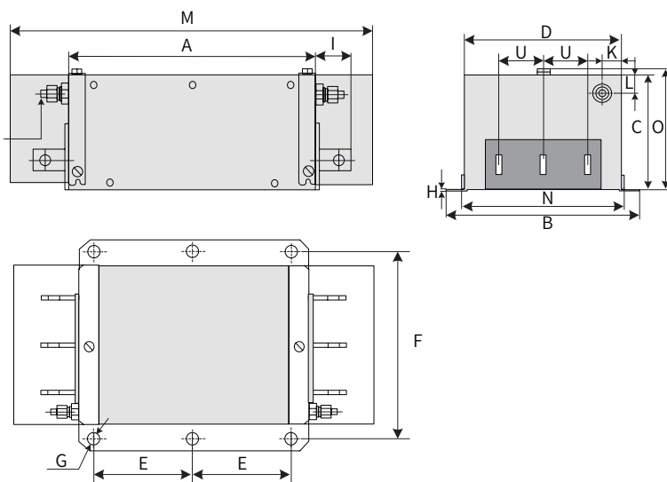
Рис. 6-13 Размеры фильтра Schaffner серии FN 3359 150 - 2500 A (в мм)
