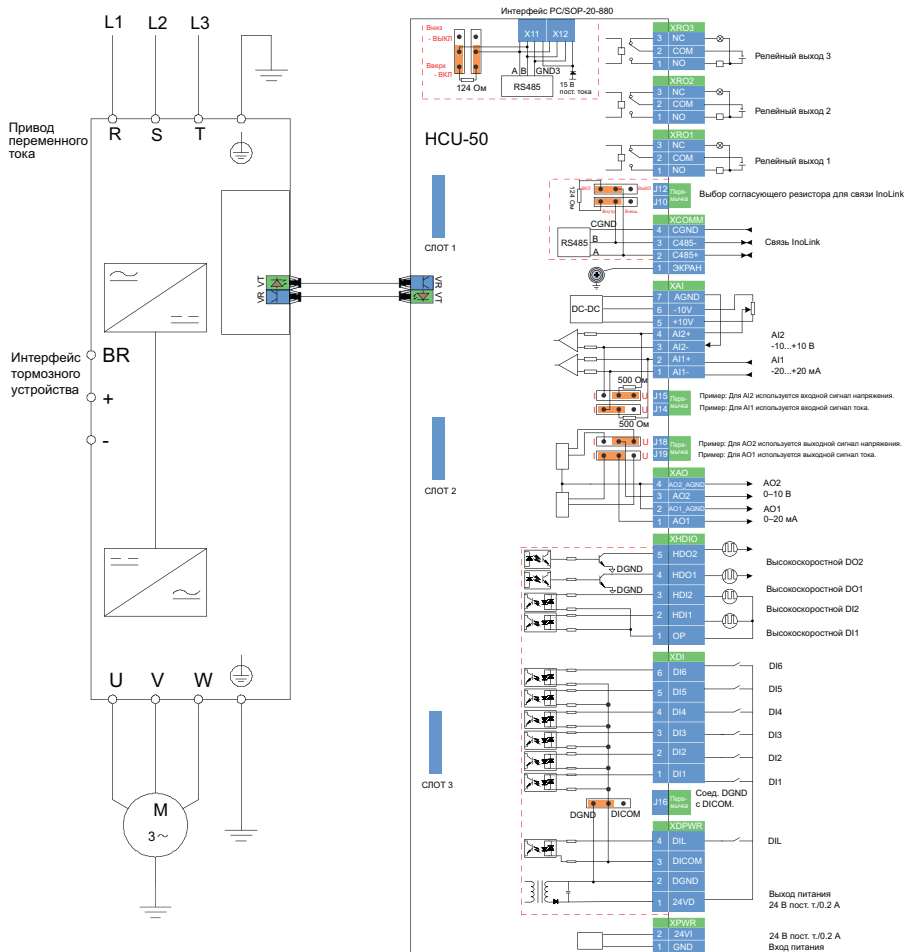
Рис. 3-12 Электромонтаж приводов переменного тока в конструкциях T10 - T12
