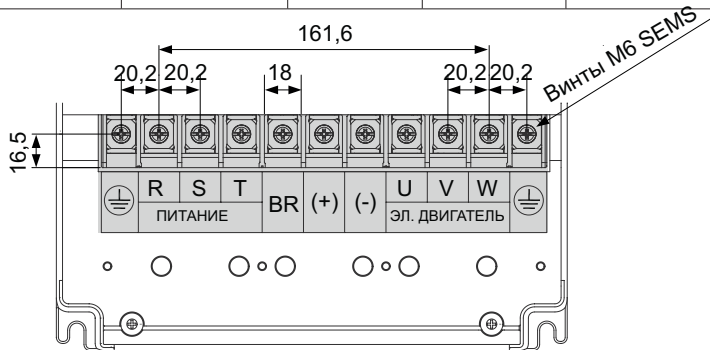
Рис. 3-28 MD880-01S-0078-4-B/MD880-01S-0094-4-B
