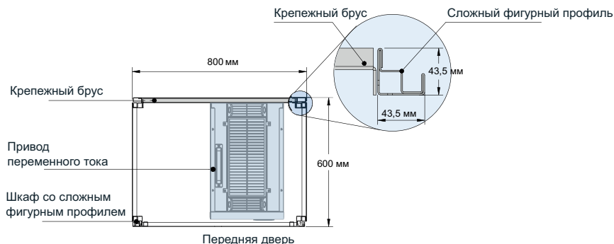
Рис. 2-13 Вид сверху на конструкции T10 - T12 в шкафу
