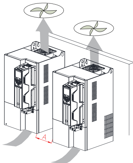
Рис. 2-5 Монтаж нескольких приводов переменного тока (тип T2–T9) в параллельной
