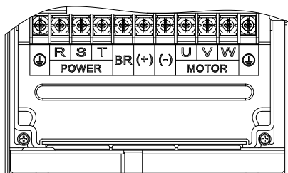
Рис. 3-14 Расположение клемм главной цепи конструкций T5 - T6
