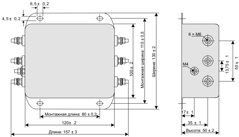
Рис. 6-18 Монтажные размеры простого ЭМС-фильтра (в мм) Табл. 6-18 Габаритные и монтажные размеры простого ЭМС-фильтра
