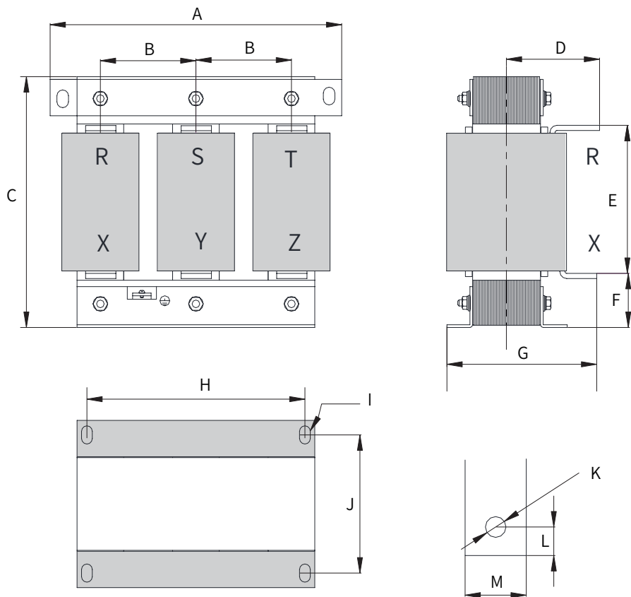
Рис. 6-8 Размеры входного реактора переменного тока 150 - 330 А
