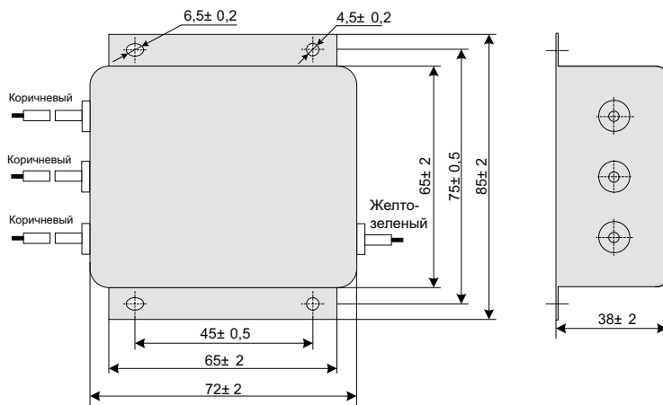
Рис. 6-20 Размеры защитного конденсатора
