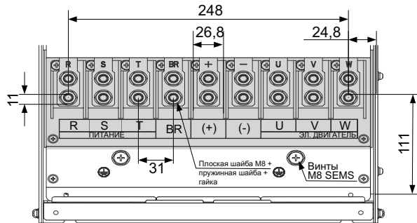
Рис. 3-29 MD880-01S-0116-4-B/MD880-01S-0149-4-B
