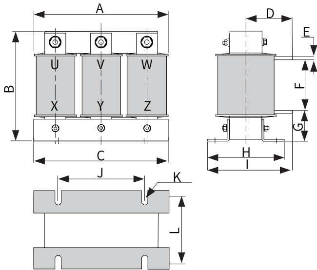
Рис. 6-28 Размеры выходного реактора переменного тока 80 - 120 A
