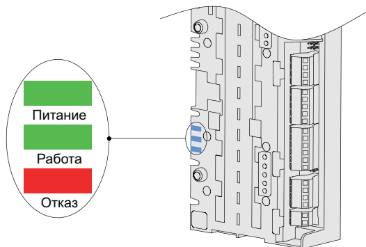
Рис. 4-5 Расположение и описание светодиодных индикаторов
