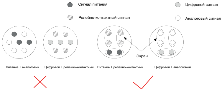
Рис. 3-5 Прокладка многожильных кабелей
