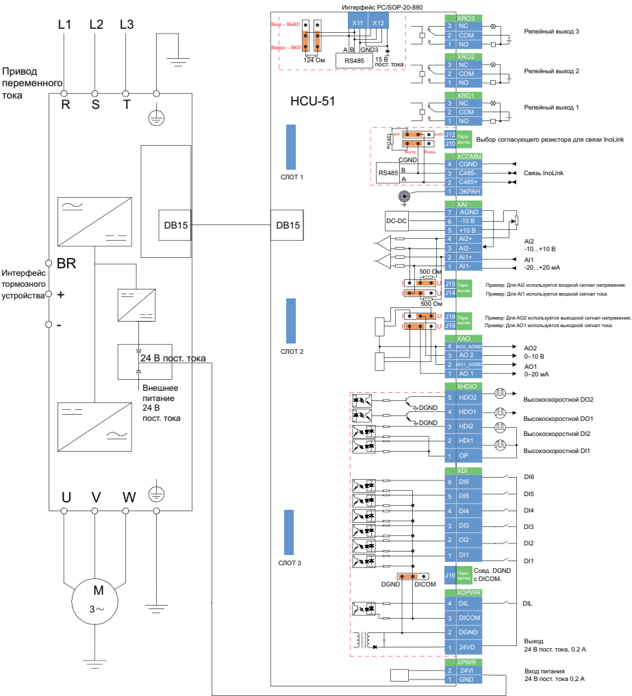
Рис. 3-11 Электромонтаж приводов переменного тока в конструкциях Т2 - Т9
