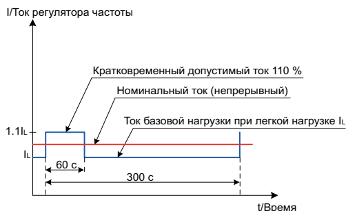
Рис. 1-5 Кривая в режиме легкой перегрузки
