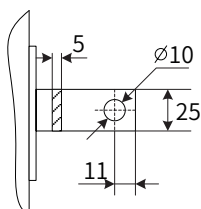
Рис. 6-16 Размеры фильтров Jianli серии 250 - 800 A (в мм)
