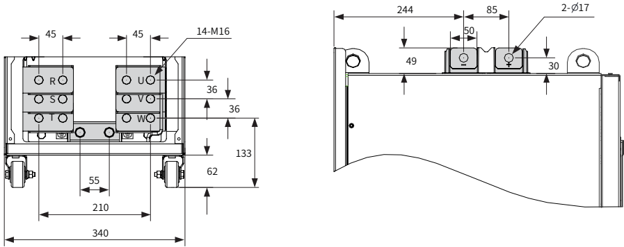
Рис. 3-40 Размеры клемм главной цепи MD880-01S-0673-4 - MD880-01S-0849-4 (без медной шины с боковым вводом и выходных реакторов)
