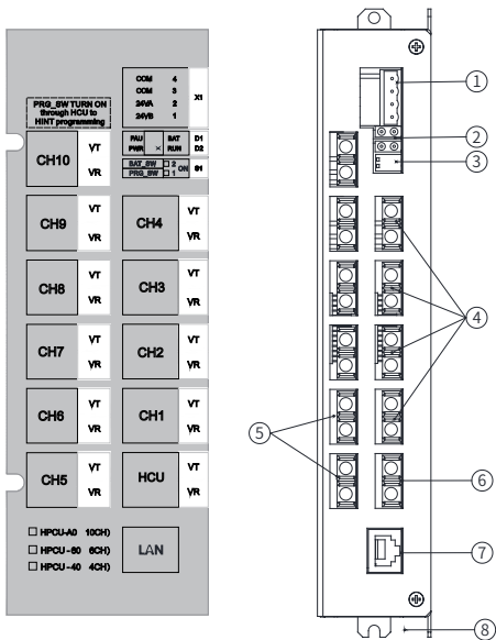
Рис. 4-7 Элементы HPCU-40/60
