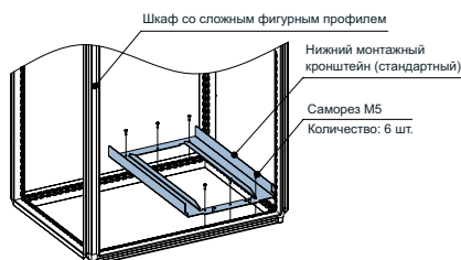
Рис. 2-15 Установка нижнего монтажного кронштейна
