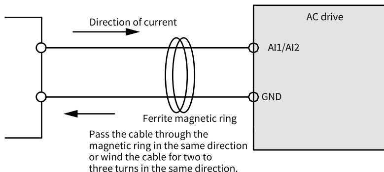
Figure 3-16 Wiring AI1/AI2
