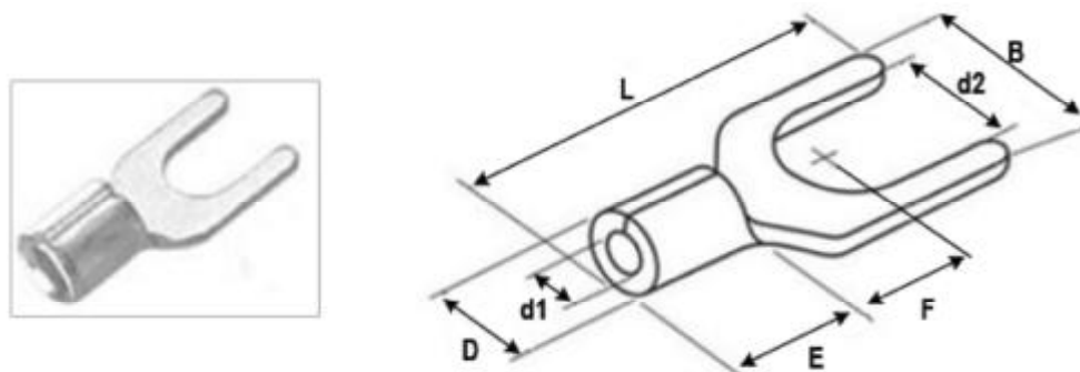
Рис. 4-8. Внешний вид и размеры рекомендуемого кабельного наконечника TNS (лопатка)
