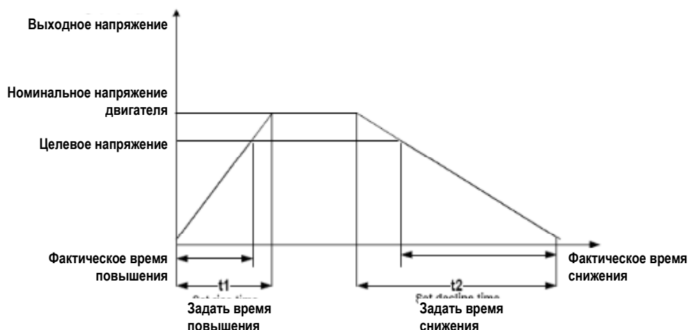
Рис. 8-5. Разделение V/F
