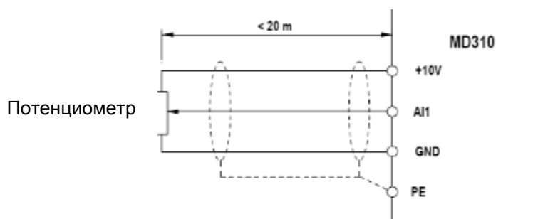
Рис. 4-9. Способ подключения для использования с аналоговым входом 1
