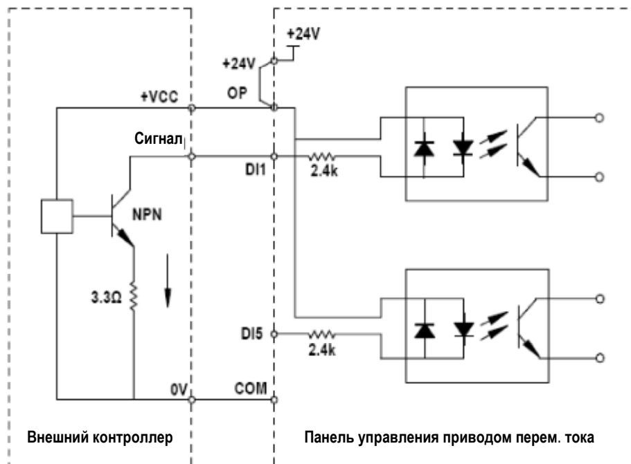
Рис. 4-10. Подключение в режиме SINK
