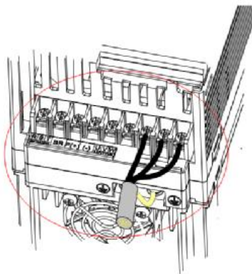
Рисунок 9-1 Заземление экранированного кабеля
