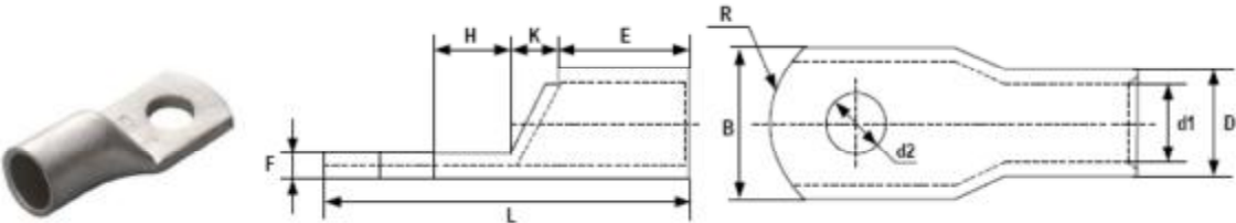
Рис. 4-6. Внешний вид и размеры рекомендуемого кабельного наконечника GTNR (кольцо)
