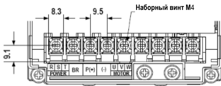
Рис. 4-2. Размеры силовых клемм MD310 - 2,2 кВт и ниже
