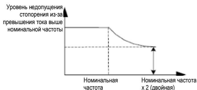
Рис. 8-7. Уровень недопущения стопорения из-за превышения тока выше номинальной частоты
