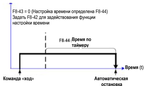
Рис. 6-14. Задание функции остановки по настройке времени
