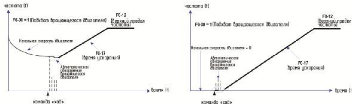
Рис. 6-10. Кривая частоты для режима подхвата вращающегося двигателя
