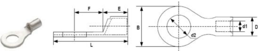
Рис. 4-7. Внешний вид и размеры рекомендуемого кабельного наконечника TNR (кольцо)
