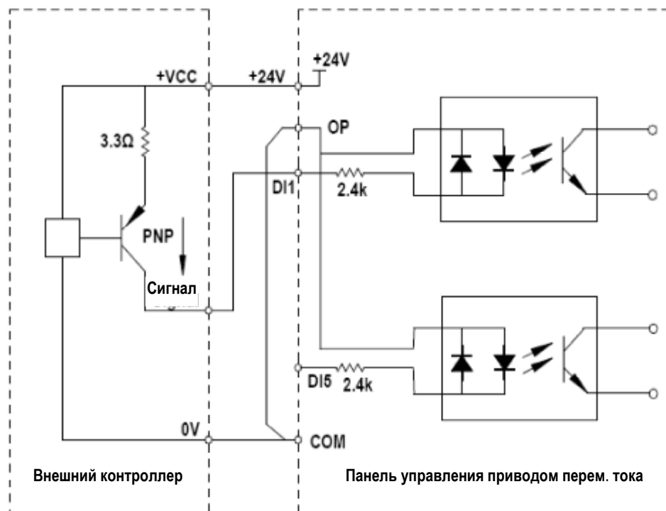
Рис. 4-11. Подключение в режиме SOURCE
