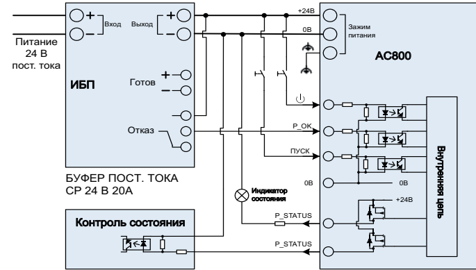
Рисунок 10 Подключение ИБП
