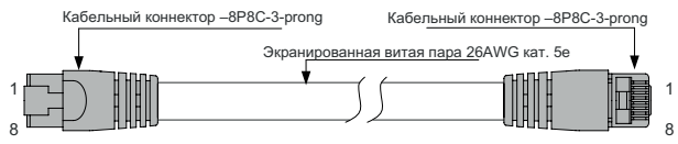
Рисунок 5 Требования к кабелю EtherCAT
