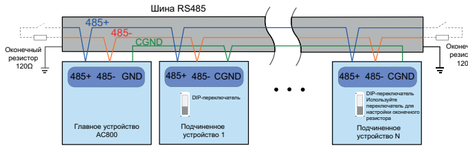
Рисунок 6 Схема подключения к каналу связи RS485
