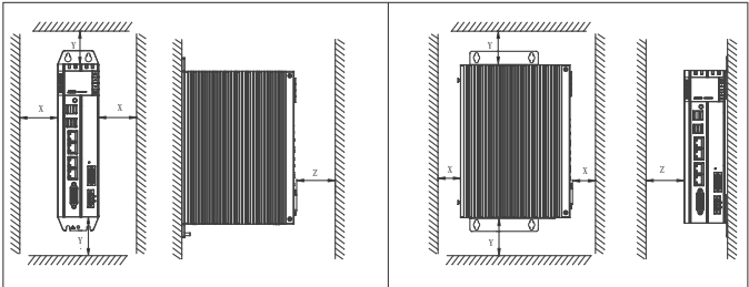
Монтаж на задний навесной кронштейн с проушинами
