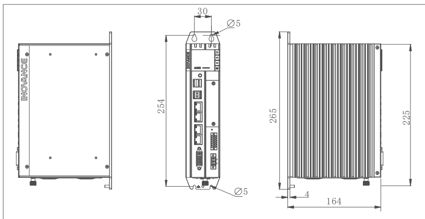
Рисунок 4-2 Монтажные размеры (задняя петля)
