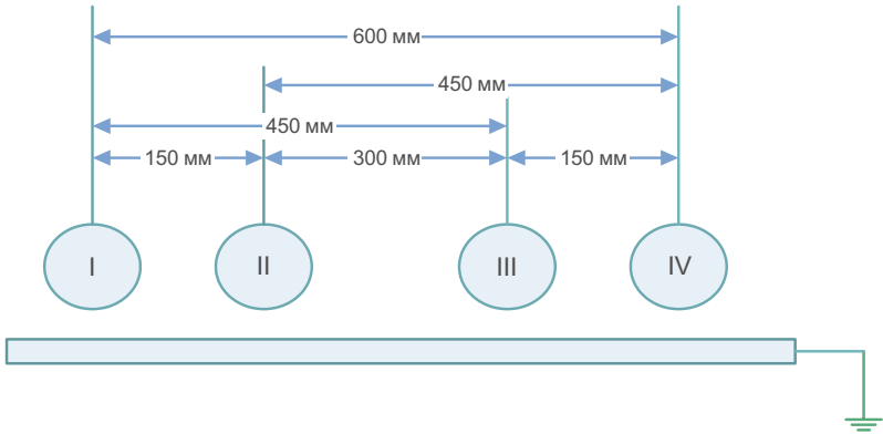
Рисунок 5-3 Расстояние между разными типами кабелей
