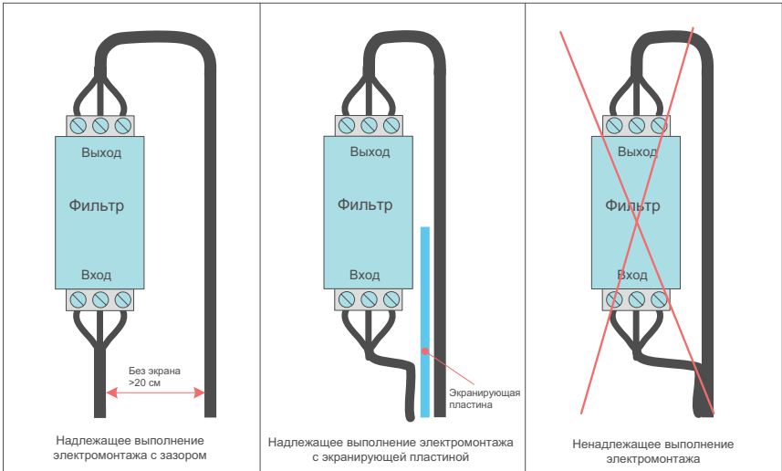
Рисунок 5-4 Установка фильтра
