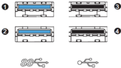
Рисунок 5-19 Порт USB
