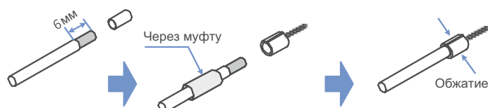
Рисунок 5-20 Подготовка кабеля со штырьковой клеммой
