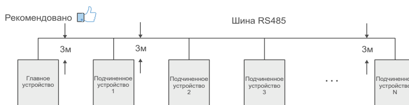
Рисунок 5-10 Ответвление
