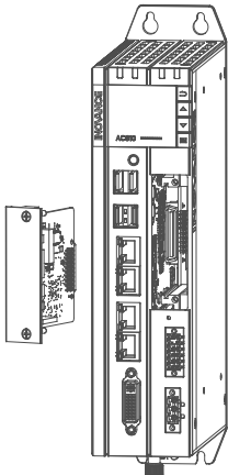
Рисунок 2-2 Слот для платы расширения
