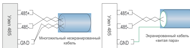
а Многожильный неэкранированный кабель
